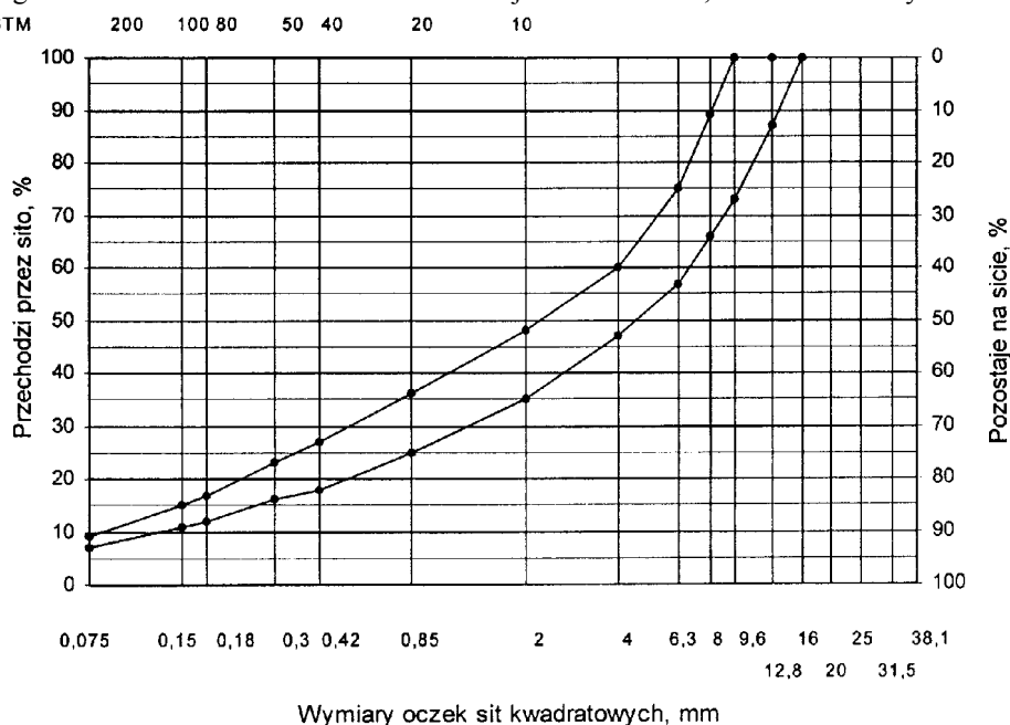
Rys. 1. Krzywe graniczne uziarnienia mieszanki mineralnej BA od 0 do 12,8 mm do warstwy ścieralnej
